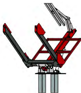
U型頂高翻滾機
